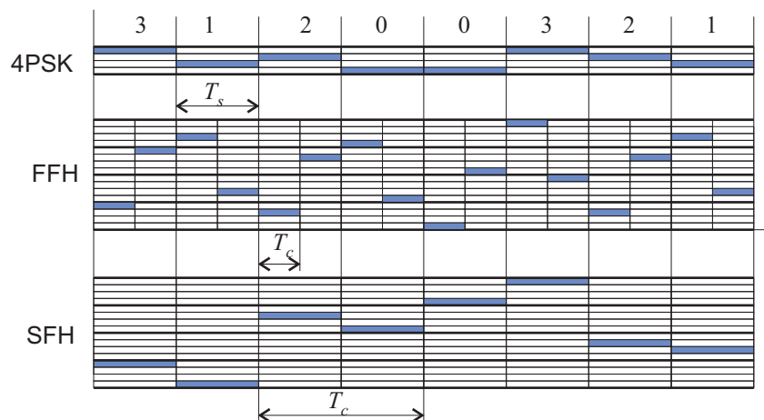
Slika 8.16 – Časovne spremembe frekvence pri 4PSK, 4PSK/SFH in 4PSK/FFH. Pri počasnem frekvenčnem skakanju se prenese več simbolov preden se spremeni frekvenca nosilca, vendar se znotraj tega frekvence spreminja zaradi frekvenčne modulacije. Pri hitrem skakanju frekvenca spreminja med prenosom enega samega simbola.
