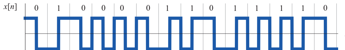
Slika 11.4 – Primer bifazne kode. Koda je enosmerno uravnorežena v okviru vsakega posameznega simbola, zato nima enosmerne komponente in tudi ne pride do problema lezenja odločitvenega nivoja
