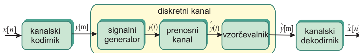
Slika 11.1 – Kanalski kodirnik preslika niz x[n] na svojem vohodu v niz y[m] , ki je bolj prilagojen prenosu po diskretnem prenosnem kanalu. Niz na izhodu kanala \hat{y}[m] kanalski dekodirnik preslika v niz \hat{x}[n] , za katerega želimo, da bi bil enak nizu x[n]
