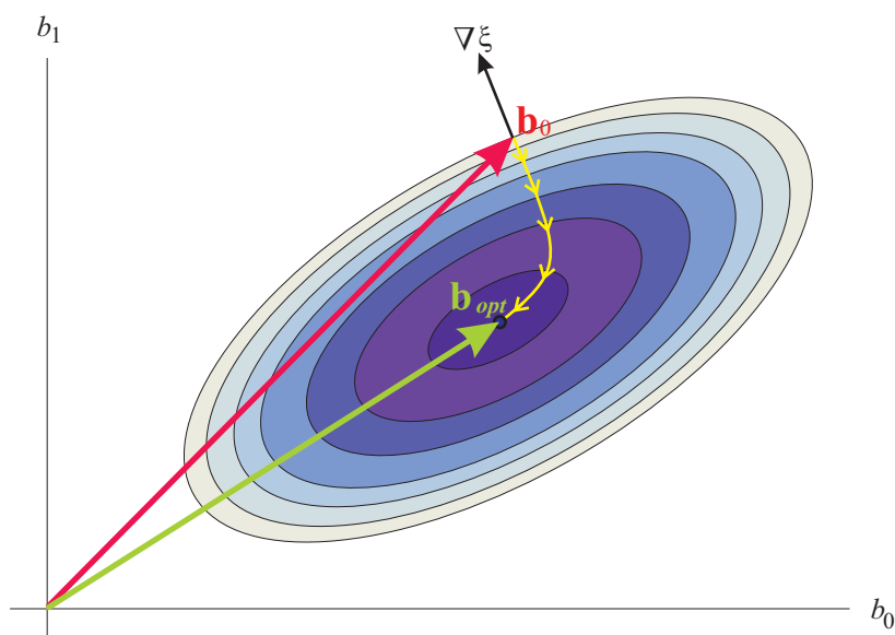
Slika 6.6 – Primer kriterijske funkcije FIR sita z dvema utežma b_0 in b_1 – pogled z vrha navzdol. Izohipse so pri dveh utežeh elipse. Gradient v vsaki točki je pravokoten na izohipso, ki gre skozi to točko. Od začetne vrednosti vektorja uteži \mathbf{b}_0 popravljamo uteži v nasprotni smeri gradienta po krivulji, ki je pravokotna na izohipse, proti optimalni vrednosti \mathbf{b}_{opt} .
