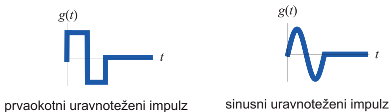
Slika 11.5 – Oblika impulzov, če na bifazno kodo gledamo kot na bipolarno kodo z uravnoreženimi impulzi
