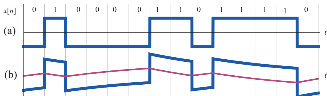
Slika 11.3 – Primer binarno kodiranega signala. Signal je enosmerno uravnovežen (a), zato nima enosmerne komponente. Pri prenosu preko transformatorja pa lahko pride pri daljših zaporedjih samih 0 ali 1 do lezjenja odločitvenega nivoja (b).
