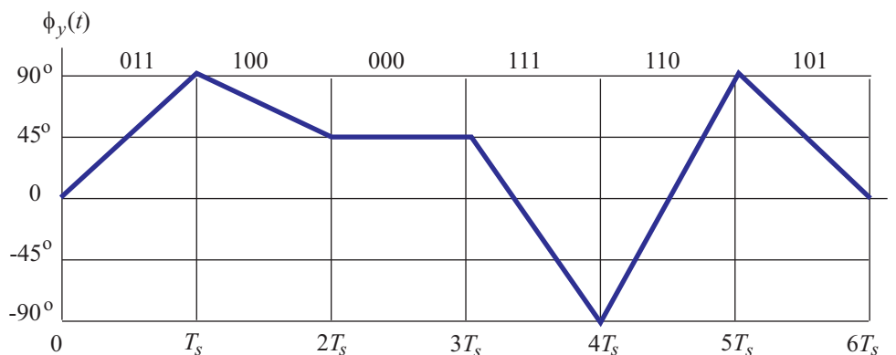
Slika 8.8 – Kadar so prehodi faze med vzorčnimi trenutki linearni, dobimo pri diferencialnem kodiranju za vsak vhodni simbol drugačen naklon, oziroma drugo frekvenco. Diferencialna fazna modulacija je zato v resnici frekvenčna modulacija oziroma FSK (Frequency Shift Keying).
