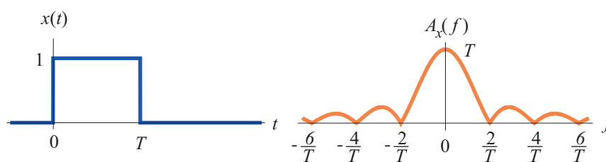
Slika 2.11 – Amplitudni spekter pravokotnega impulza. Spekter ima pri frekvenci 0 vrednost T in prvo ničlo pri frekvenci 2/T . Če manjšamo T , se amplituda zmanjšuje, frekvenčno področje pa se širi.
