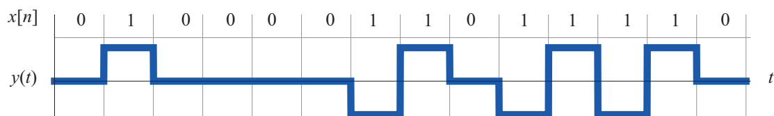
Slika 11.7 – Pri AMI kodi se predznak simbola 1 izmenjuje, zato je sprotna digitalna vsota omejena. Pri dolgih zaporedjih samih 0, pa lahko še vedno pride do izgube sinhronizacije.
